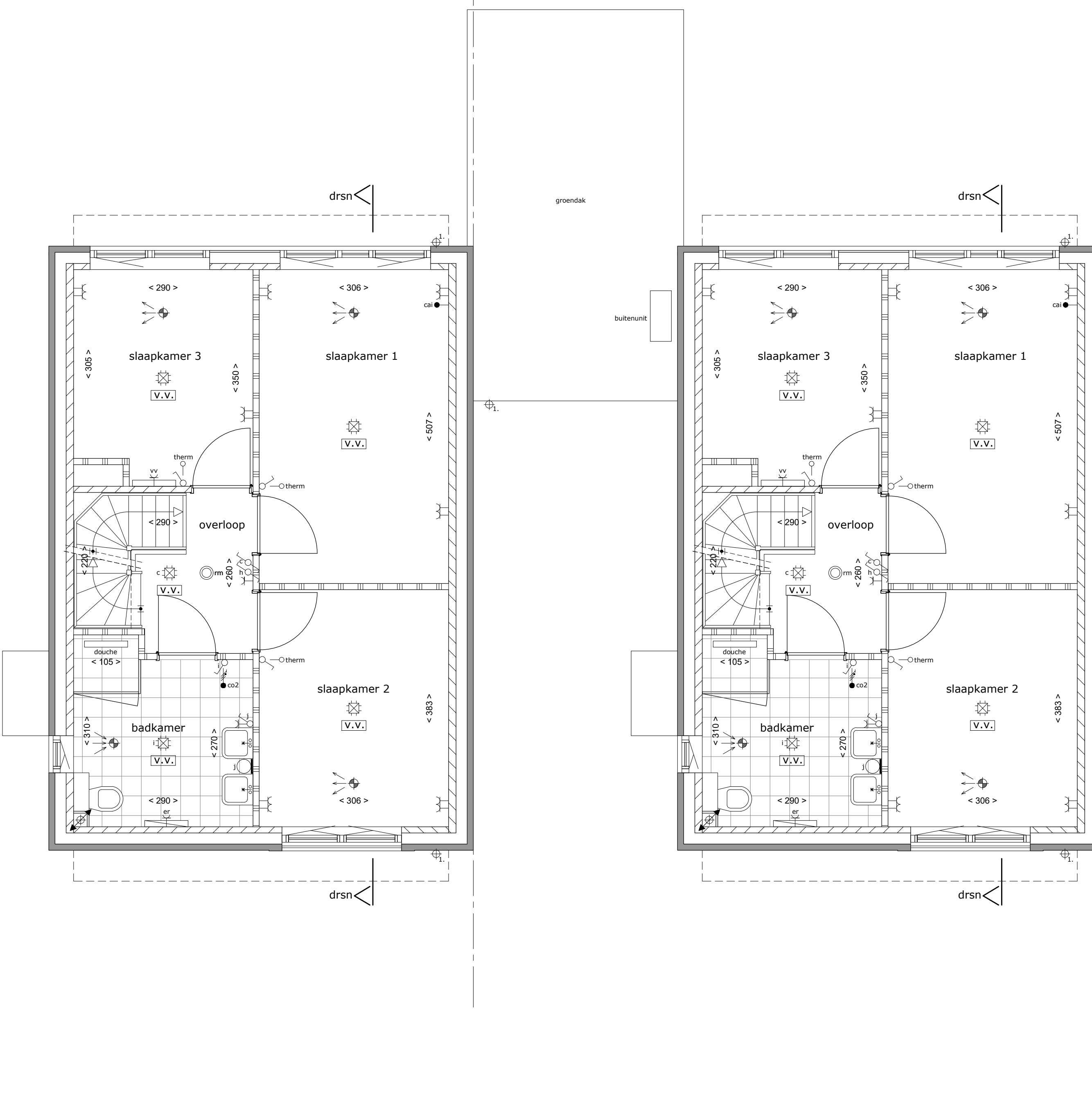
1ste verdieping schaal 1:50
