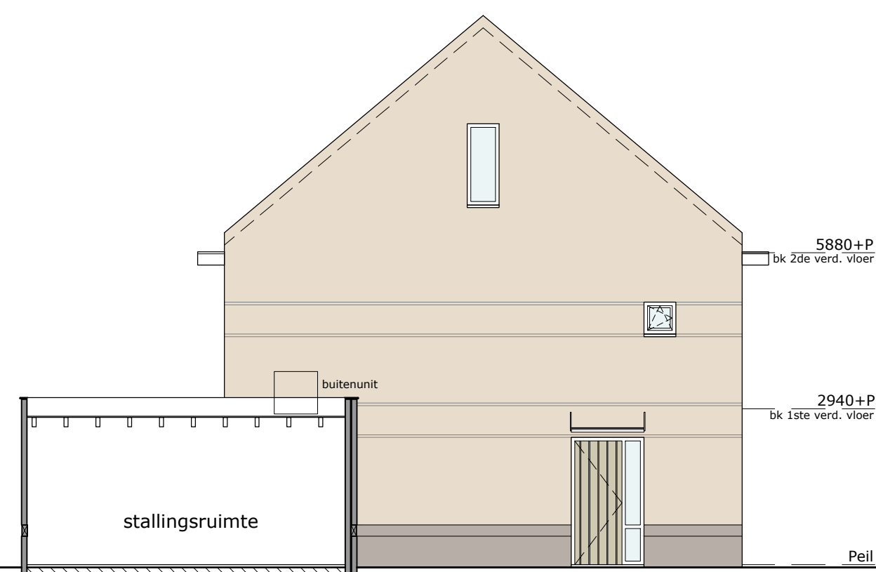
linkerzijgevel schaal 1:100
