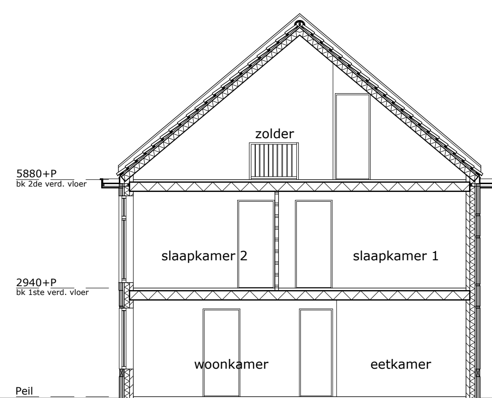
doorsnede schaal 1:100
