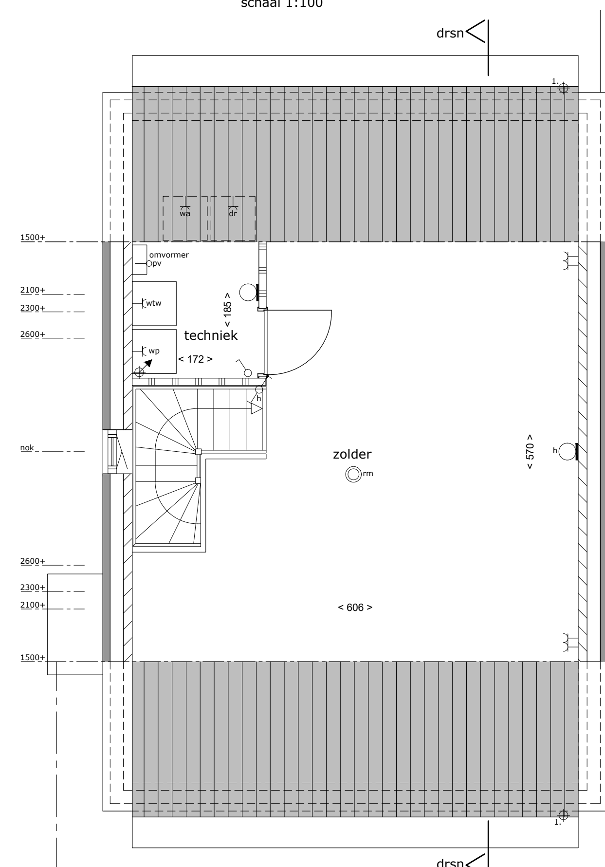
2de verdieping schaal 1:50
