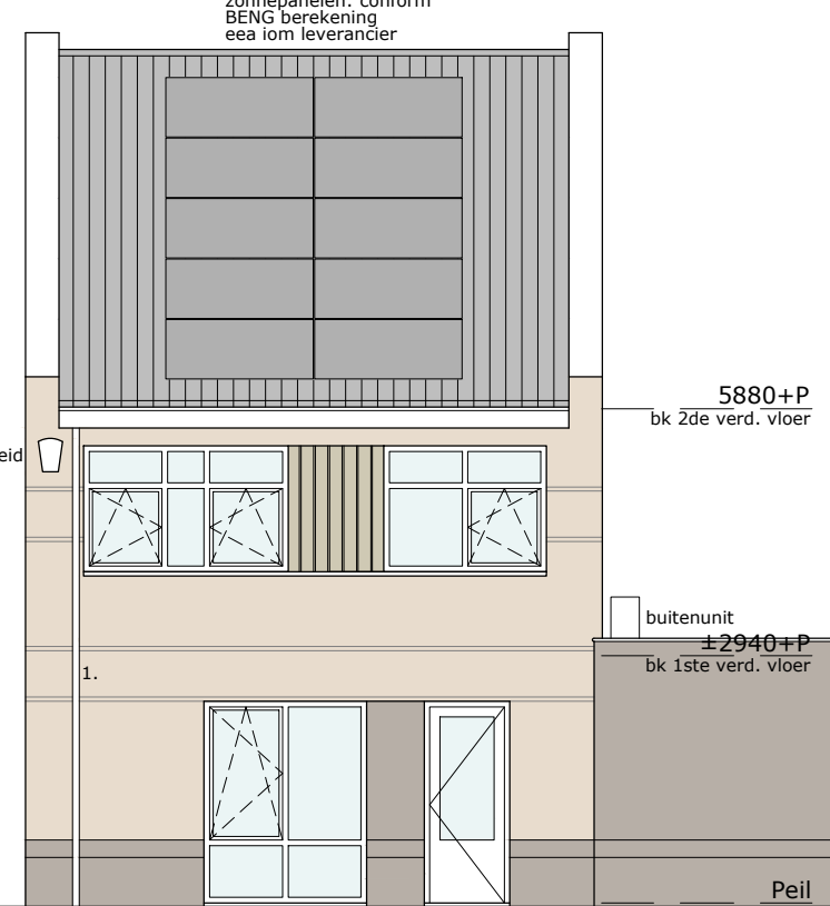
achtergevel schaal 1:100
